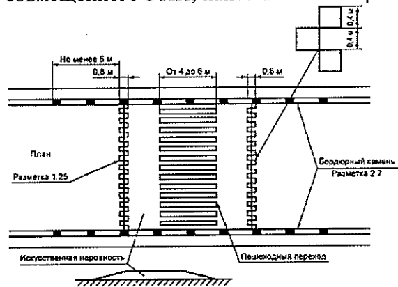
Рисунок 4 - Пример нанесения разметки 1.25 и 2.7 при устройстве ИН
